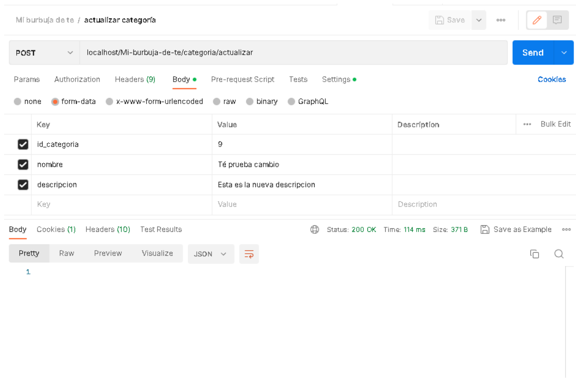
Ilustración 44: Postman para modificar categorías
