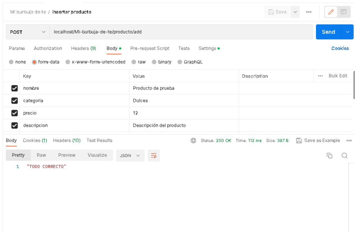
Ilustración 46: Postman para crear productos
