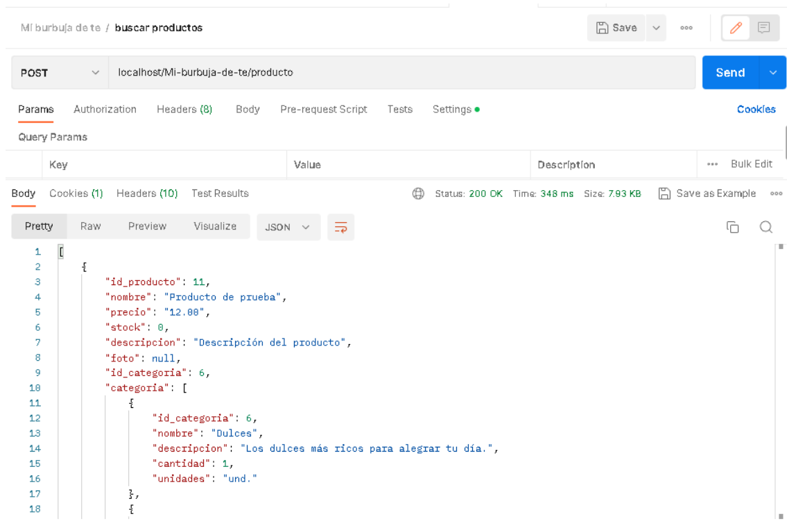
Ilustración 45: Postman para consultar productos
