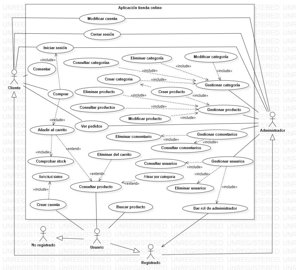
Ilustración 1: Diagrama de casos de uso
