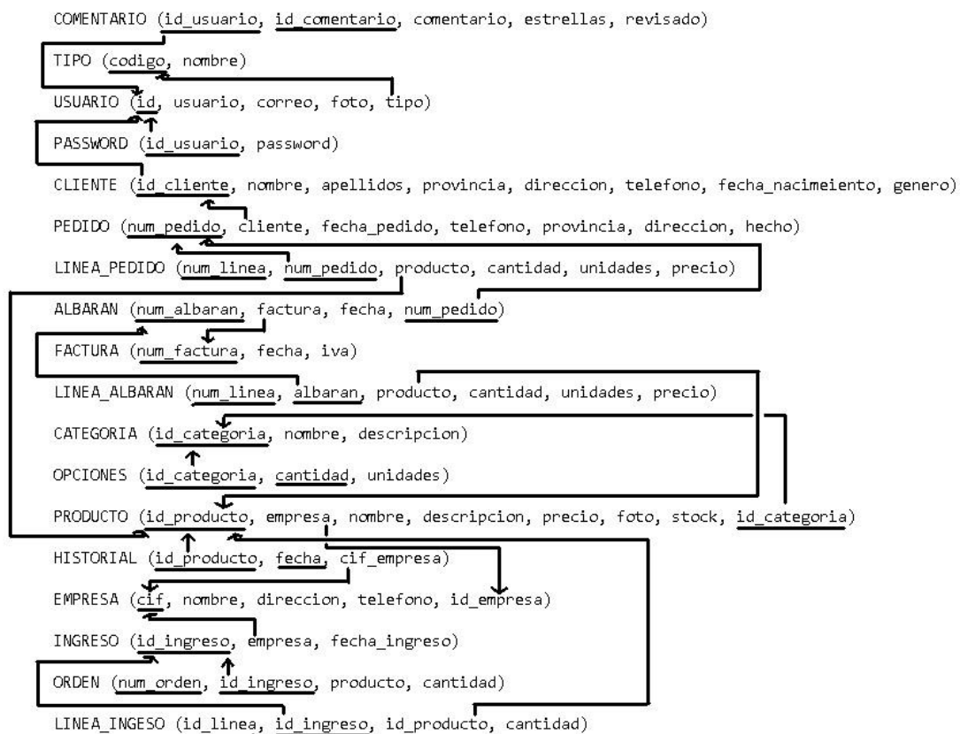
Ilustración 13: Modelo relacional
