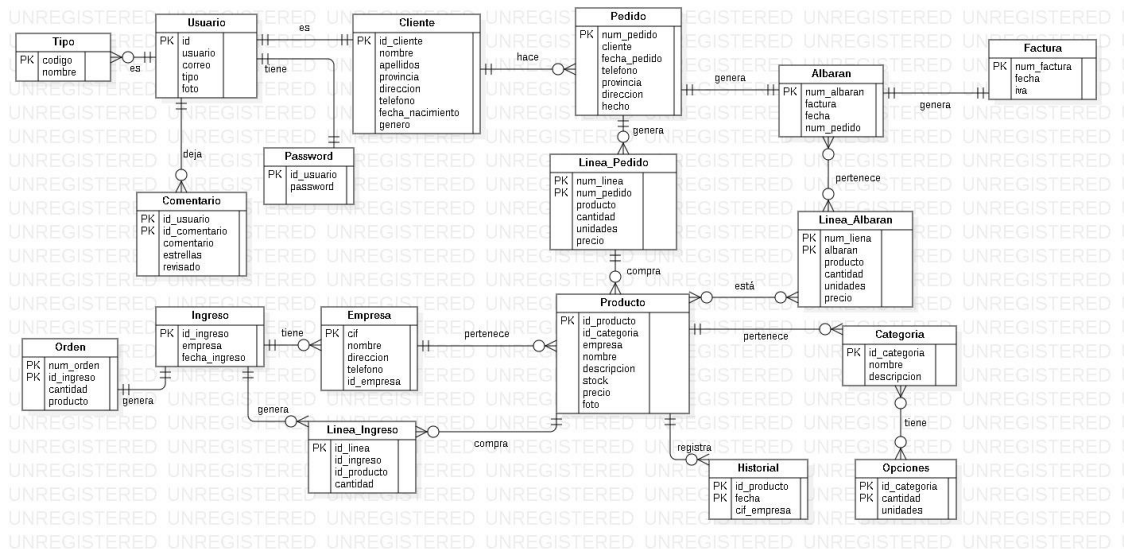
Ilustración 3: Modelo Entidad-Relación
